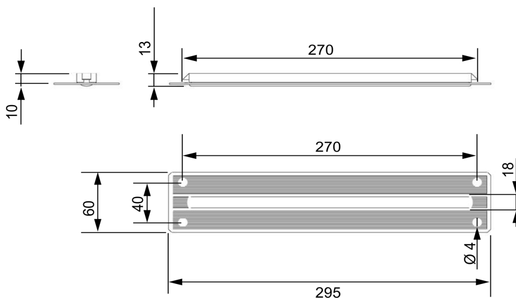
Obr. 1: Rozměry svítidla
