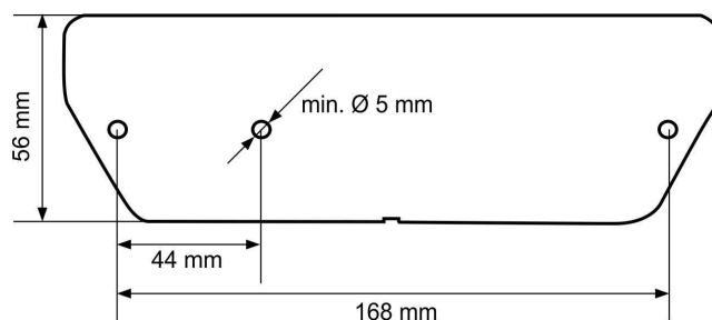
Obr. 2: Rozměrový náčrt svítidla
