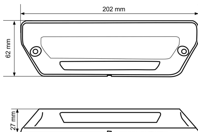
Obr. 1: Rozměry svítidla včetně gumové podložky
