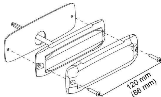
Obr. 5: Mechanické uchycení svítidla
