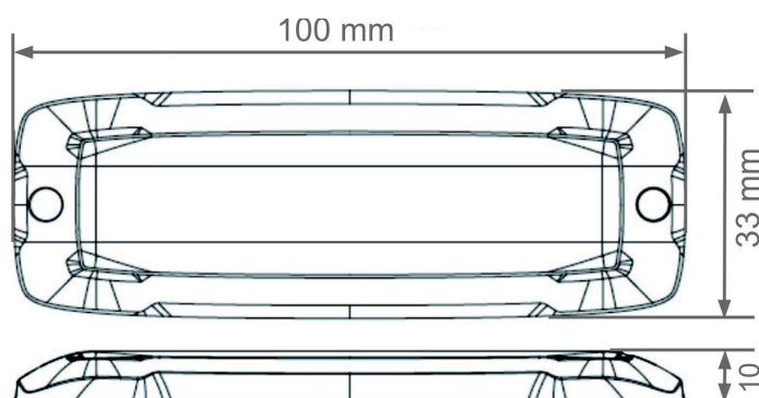
Obr. 3: Rozměry výrobku LED (x) 42-XT6 R65
