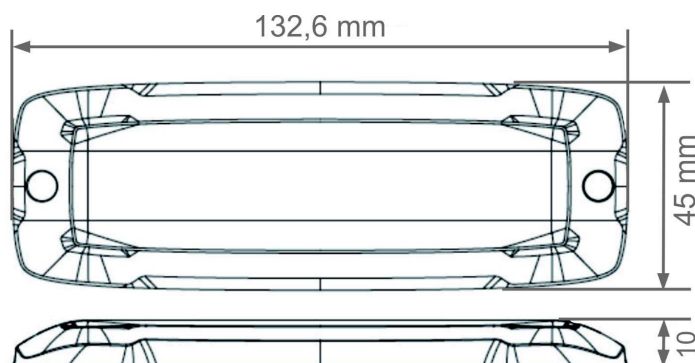
Obr. 1: Rozměry výrobku LED (x) 42-XT12 R65
