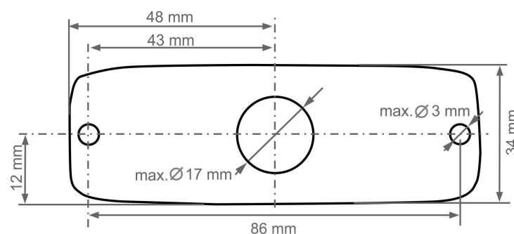
Obr. 2: Rozměrový náčrt výrobku LED (x) 42-XT12 R65
